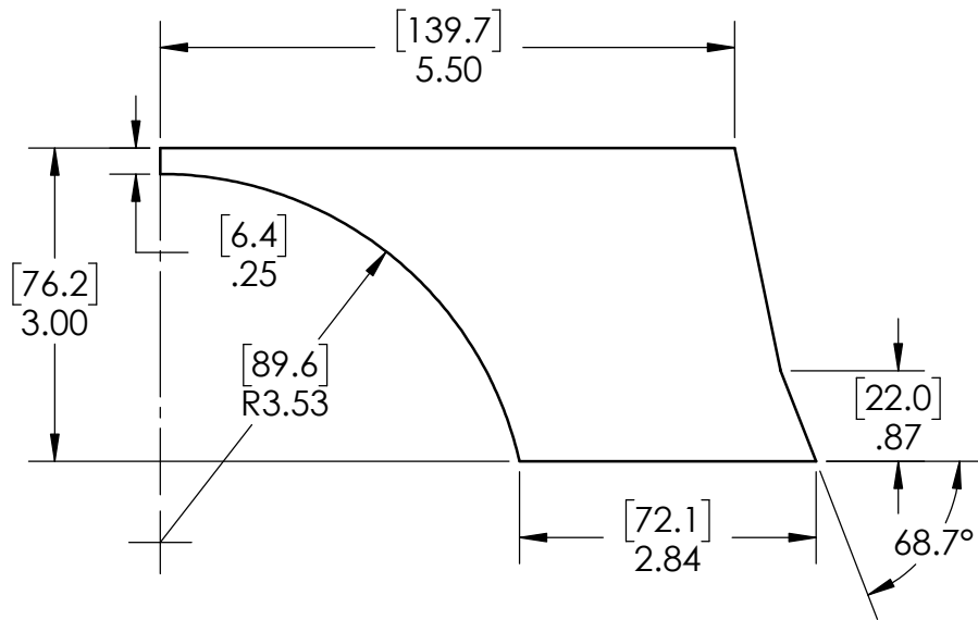
FLAT GUSSET 2 RQD PER AXLE
